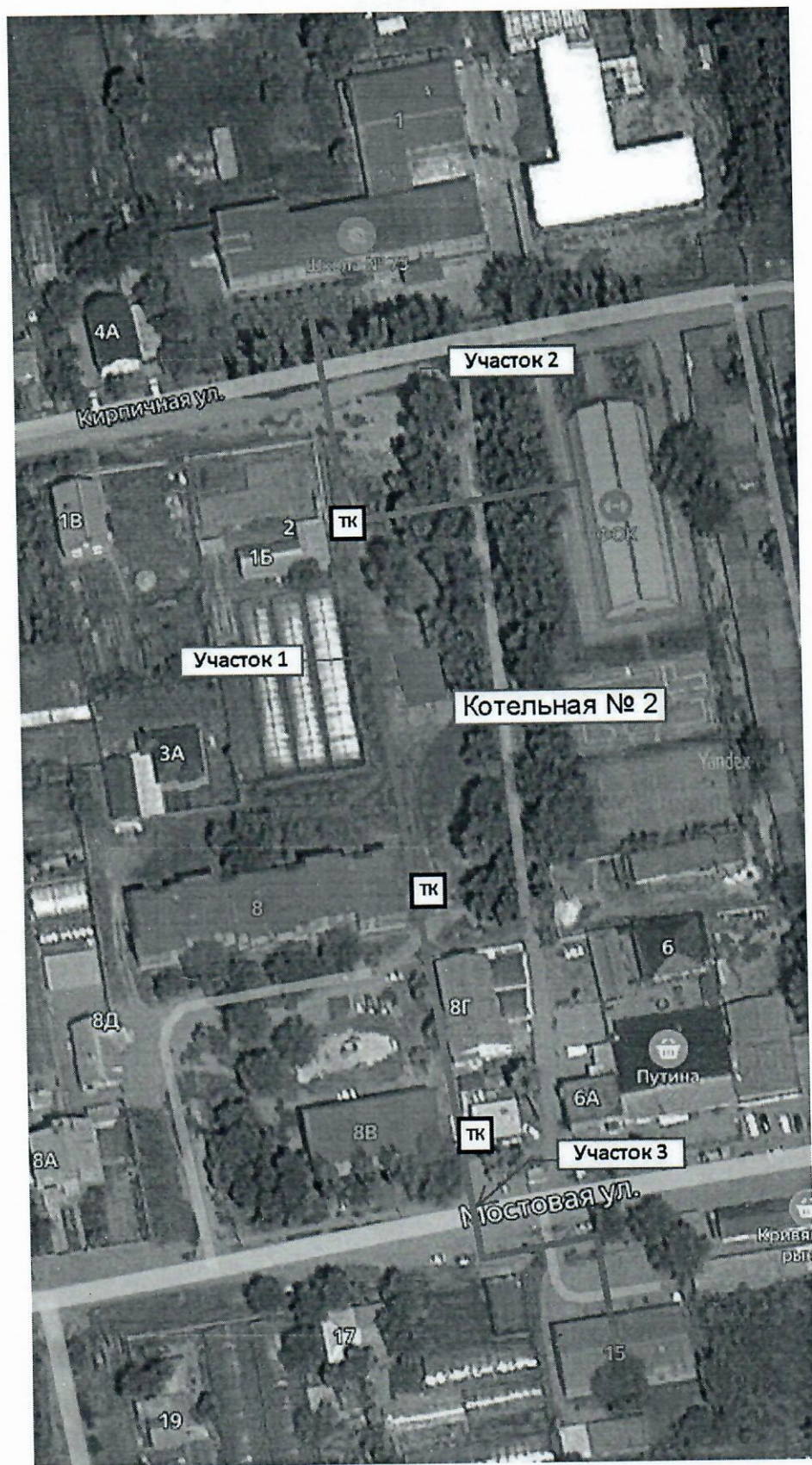
Рис. 2 – Схема тепловых сетей от котельной № 2 ст. Кривянской ул. Кирпичная д. 1Г
