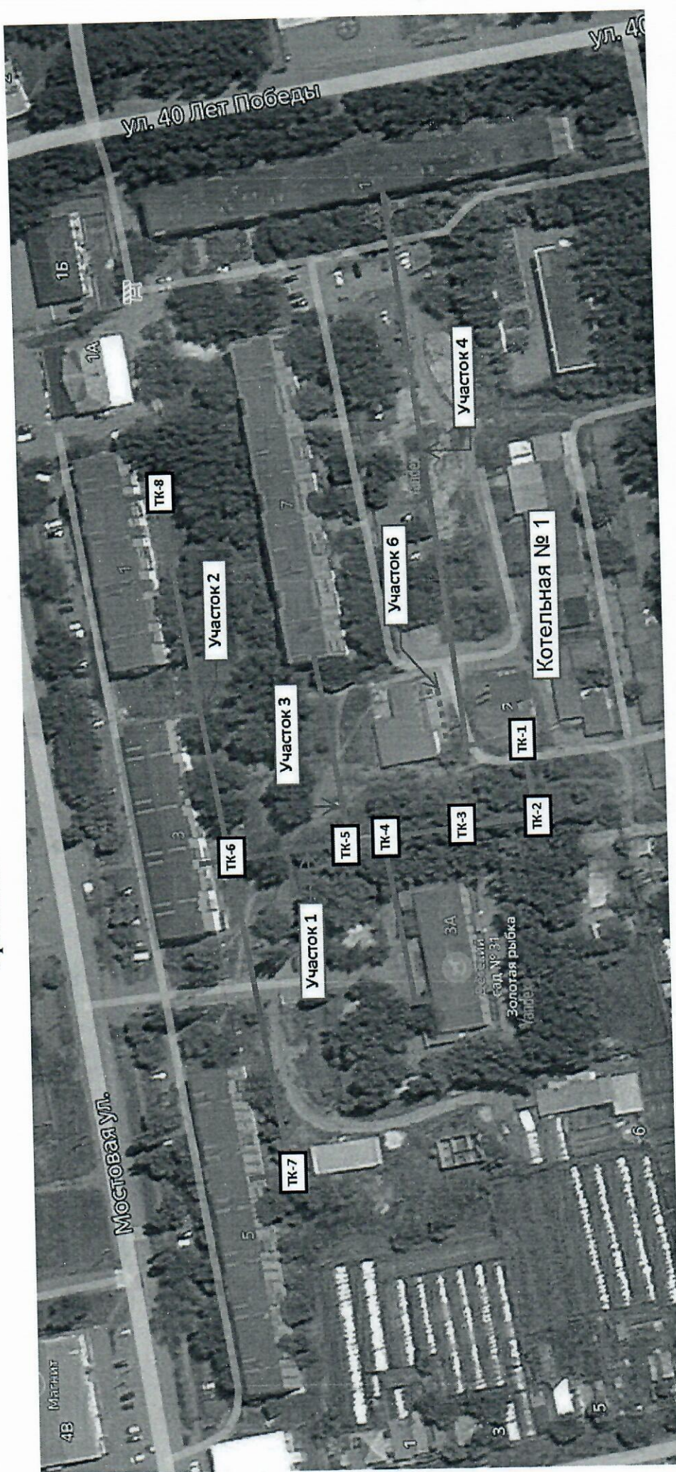
Рис. 1 – Схема тепловых сетей от котельной № 1 ст. Кривянской ул. Октябрьская д. 2Г
